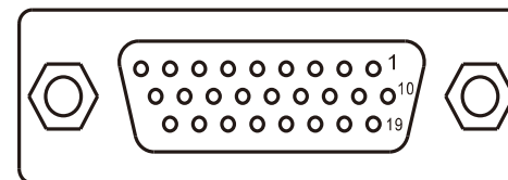
控制信号引脚排列
